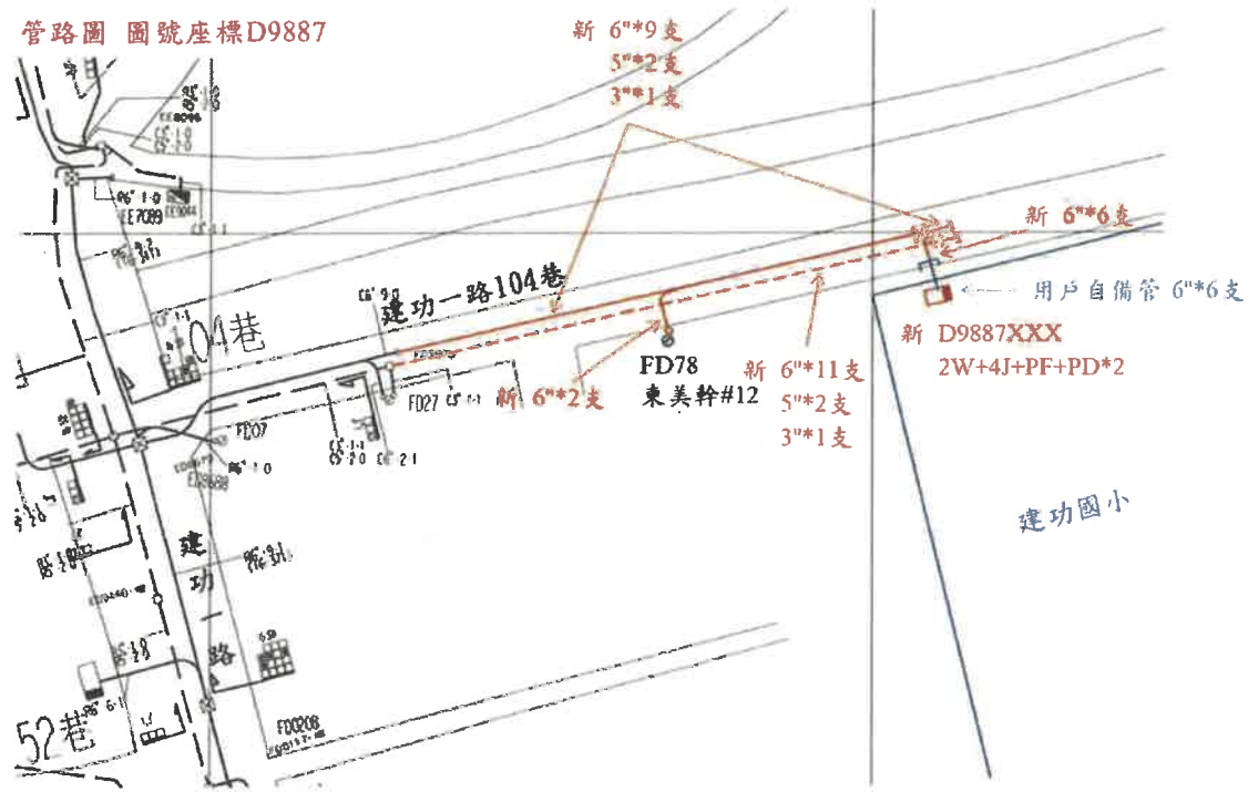
電氣圖 圖號座標D9887
